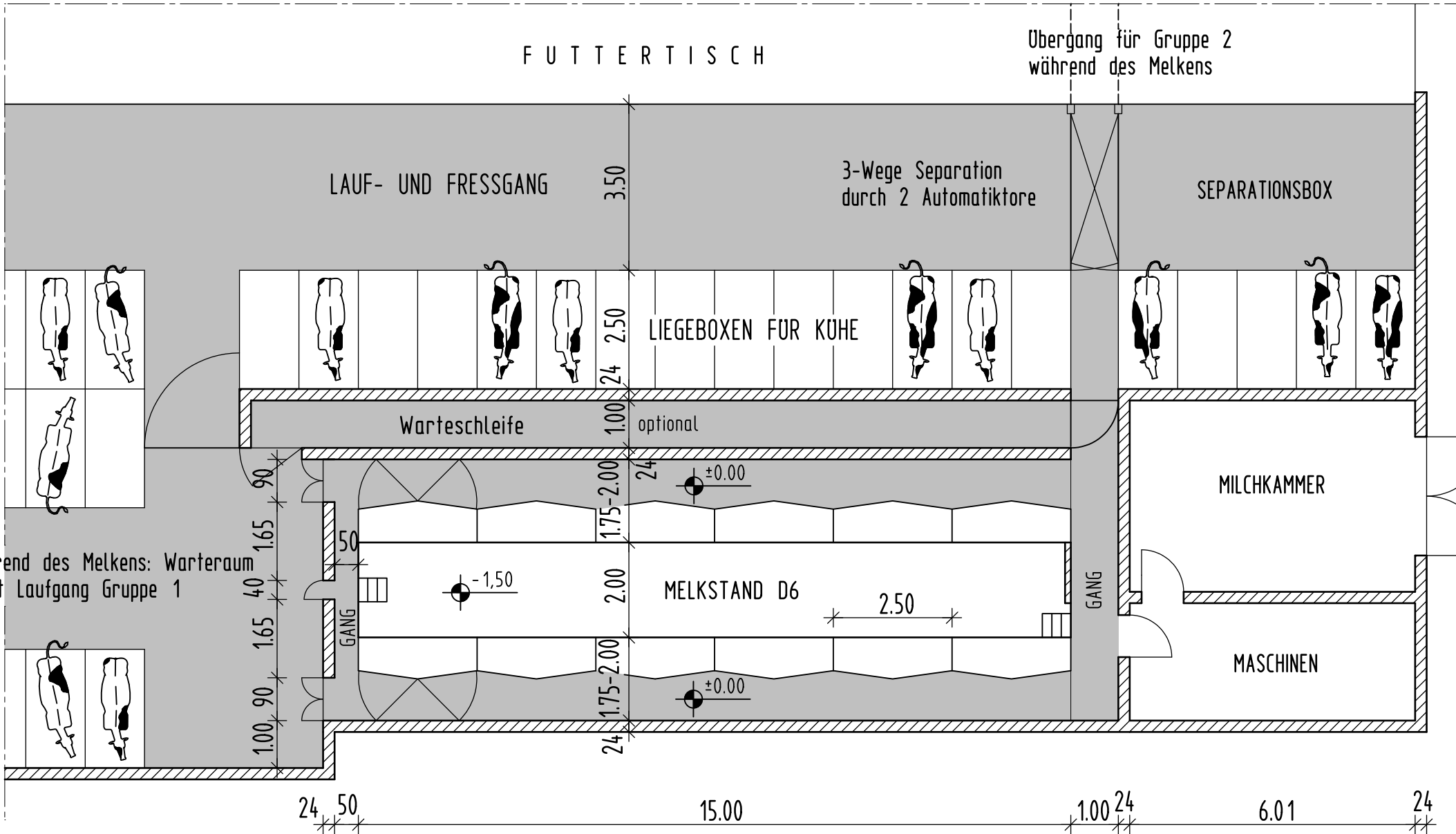
GRUNDRISS TANDEMELKSTAND DOPPEL 6
